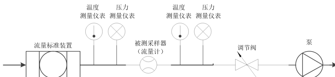
图2 流量校准示意图
