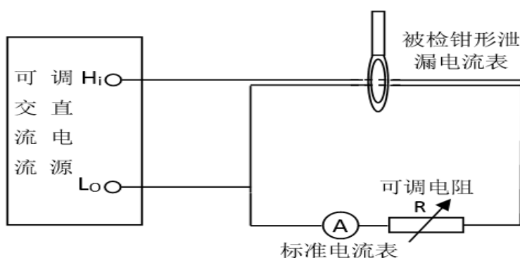
图4 负载电流影响检定示意图
