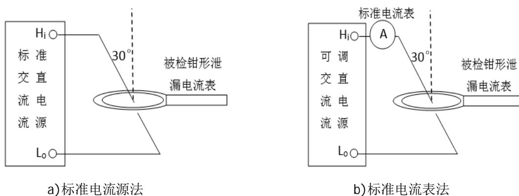
图3 电流角度影响检定示意图
