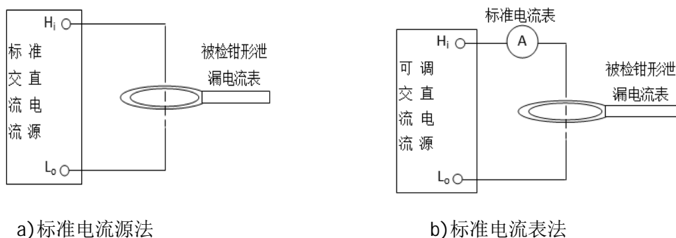
图1 检定原理示意图
