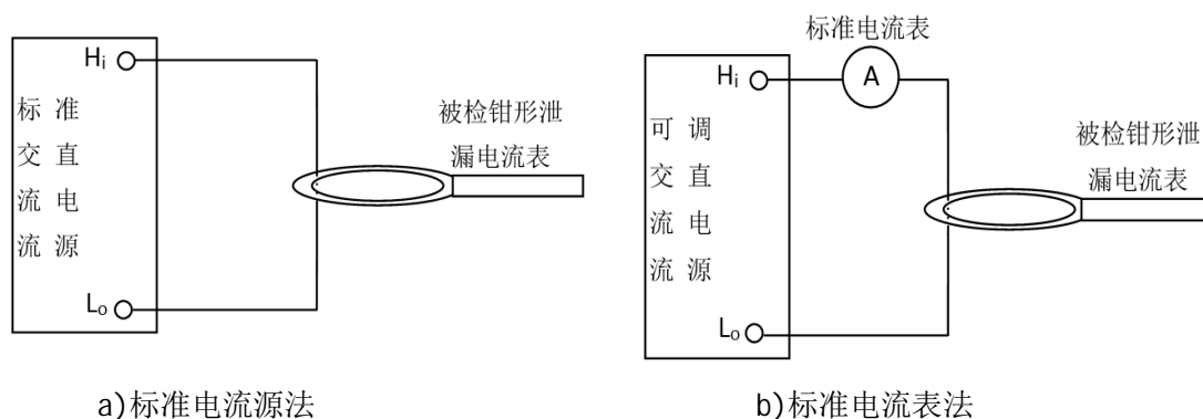
图 2 电流位置影响接线示意图
